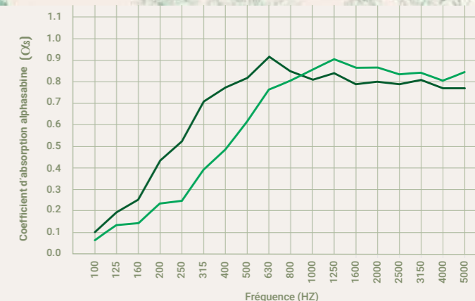
— tableau Addenda 37 mm montage au sol — tableau Addenda 64 mm montage au sol Courbe extraite du rapport du FCBA n° 404/18/1231/ du 11/07/2018 (normes NF EN ISO 354 et NF EN ISO 11654) Courbe extraite du rapport du FCBA n° 404/18/123/2, 11/07/2018 (normes NF EN ISO 354 et NF EN ISO 11654)
